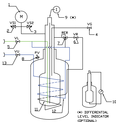
P&ID Serbatoio Mod. CRIOGAS 25 con VS1 configurata a 25 bar.
